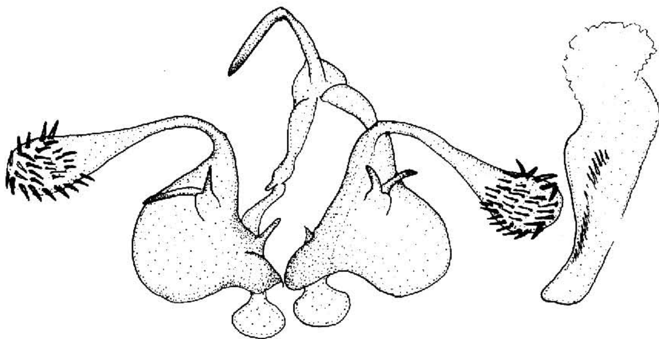
图 409 柔研夜蛾 Aletia placida (Butler) ♂ 外生殖器
